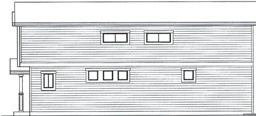
RIGHT ELEVATION
