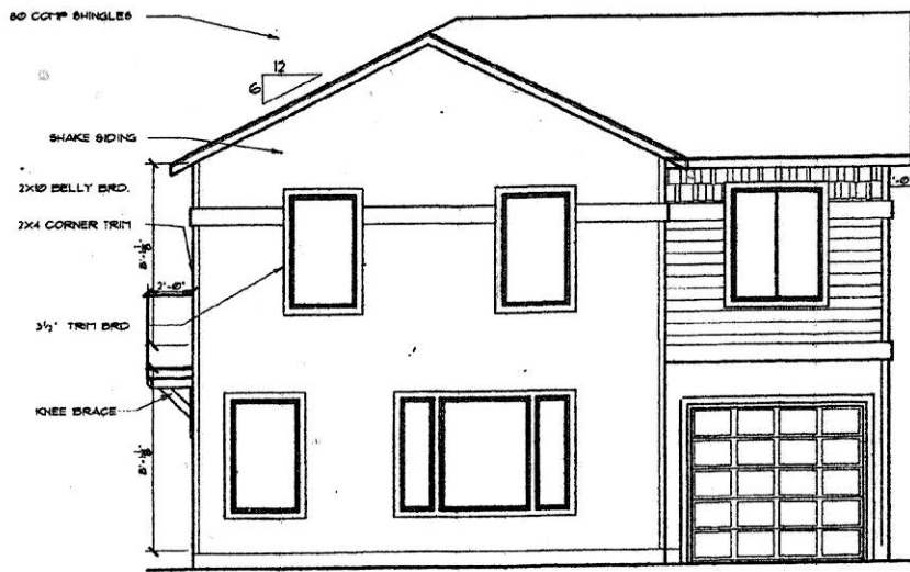
RIGHT ELEVATION
